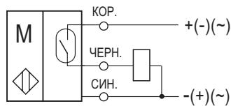
Схема подключения нагрузки
